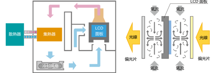
NEC 獨特 LCD 面板冷卻方法
